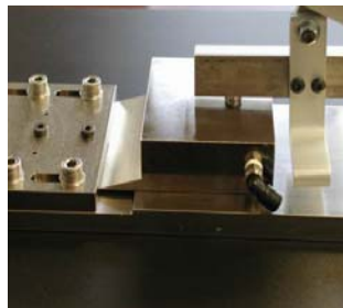
Calibración a cero con Yunque de Dispositivo de Inspección por Barrido
